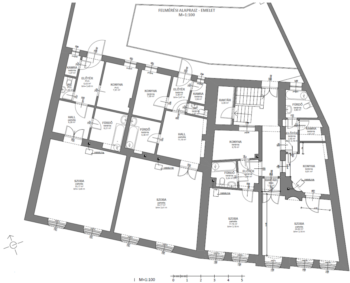
emeleti alaprajz
