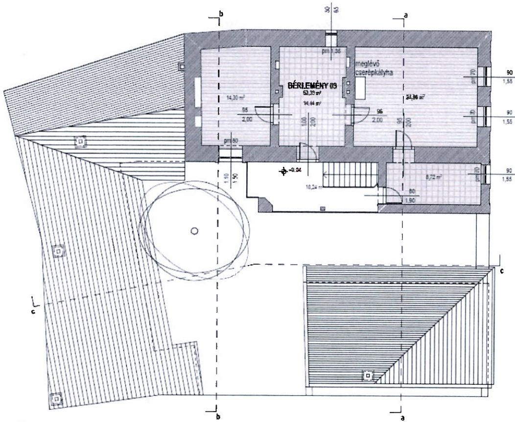
emeleti alaprajz
