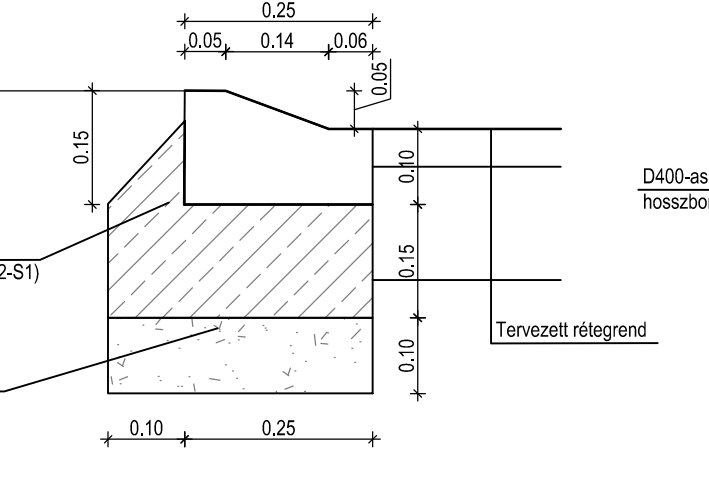
Előregyártott rácsos folyóca M=1:10
