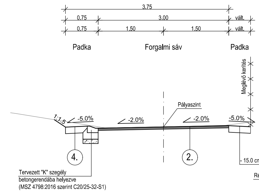
Kapubehajtó 0+011.55 - 0+042.20 km sz. M=1:50
