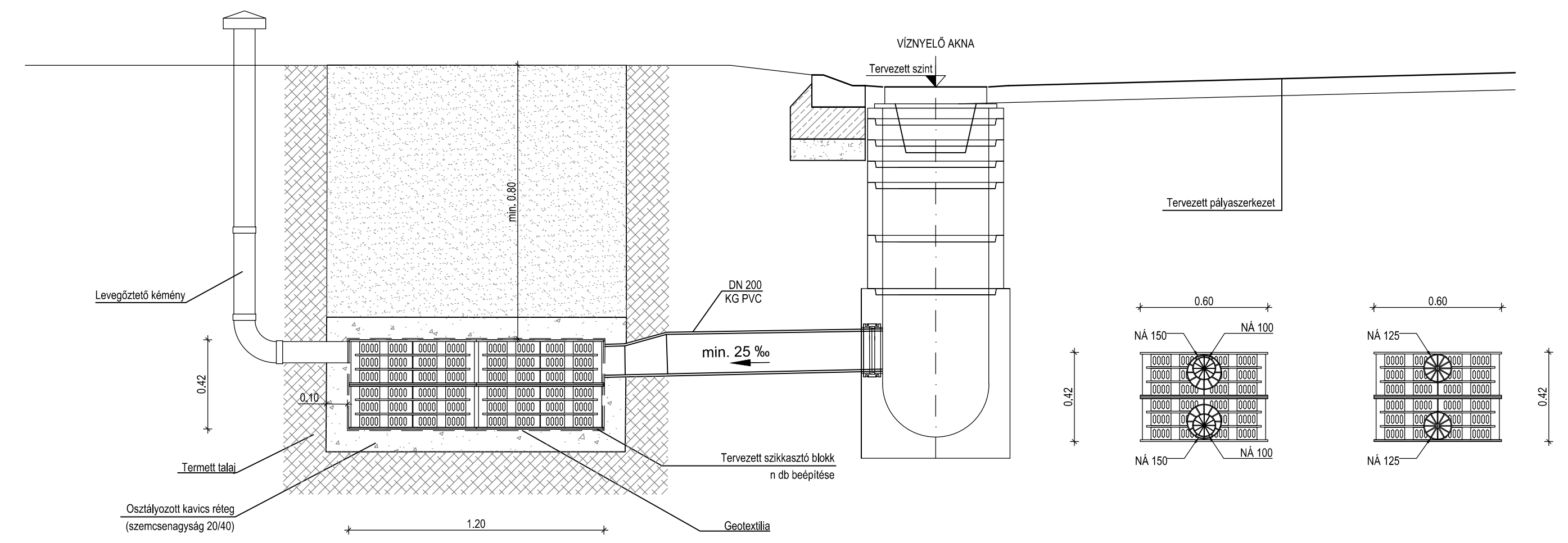
Víznyelőakna bekötése szikkasztó blokkba részletraaj M=1:20
