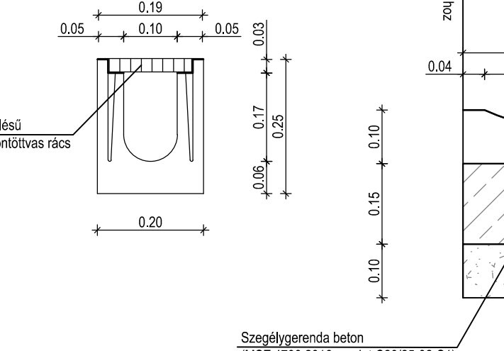
Előregyártott útpadka folyóca elem M=1:10
