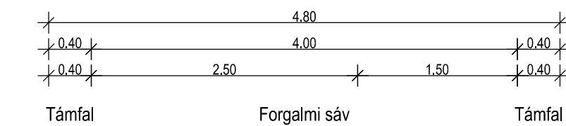
Kapubehajtó 0+079.94 - 0+084.73 km sz. M=1:50
