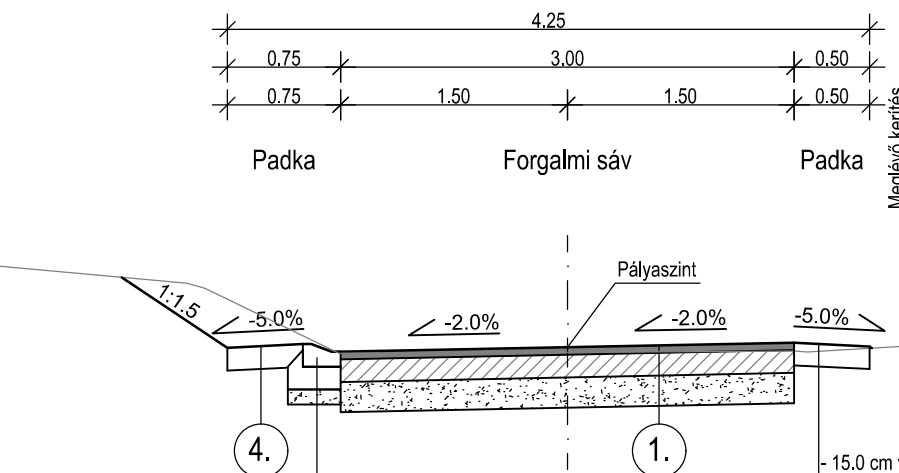
Kapubehajtó 0+058.89 - 0+072.00 km sz. M=1:50
